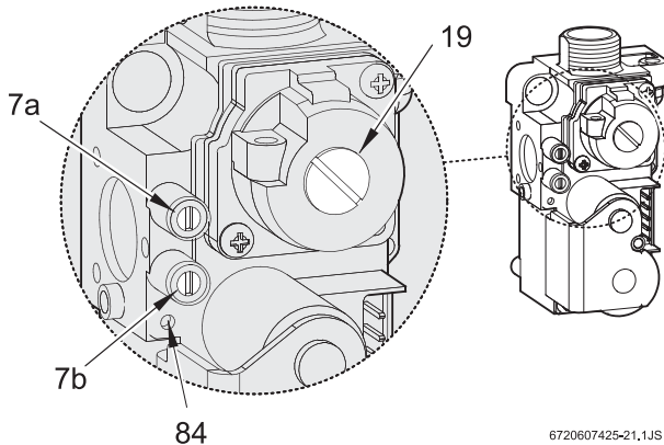
Рис. 5 Газова арматура
