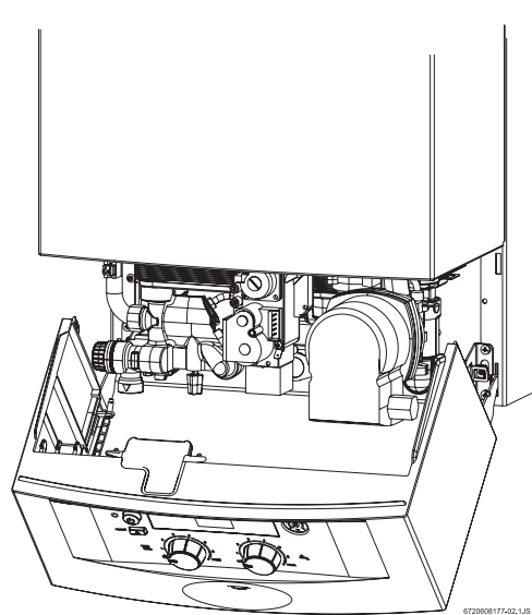
Рис. 4 Блок у сервісному положенні
